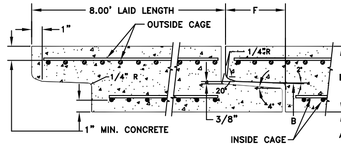
48", 54", 60", 66", 72", & 78" CLASS 3, 4, & 5
